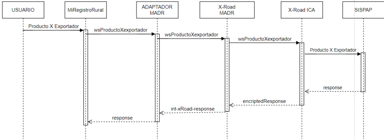
Diagrama de secuencia para consultar el servicio expuesto por ICA.
